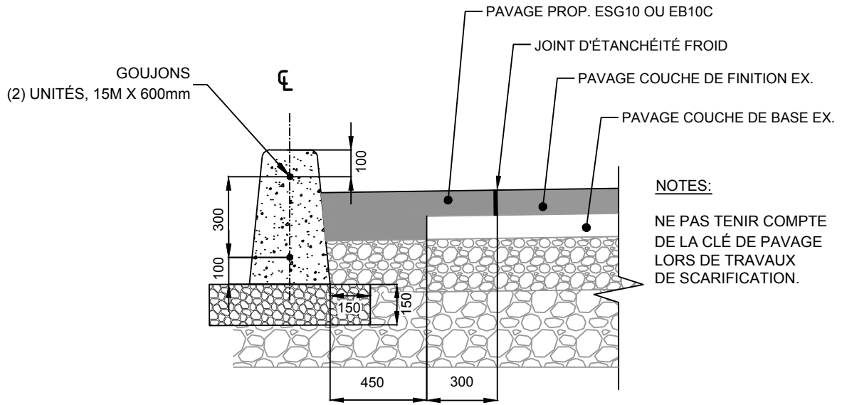
COUPE "B" : BORDURE
