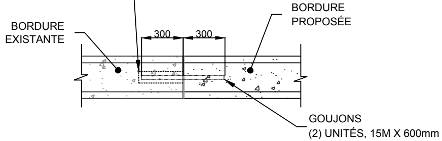
VUE EN PLAN BORDURE
