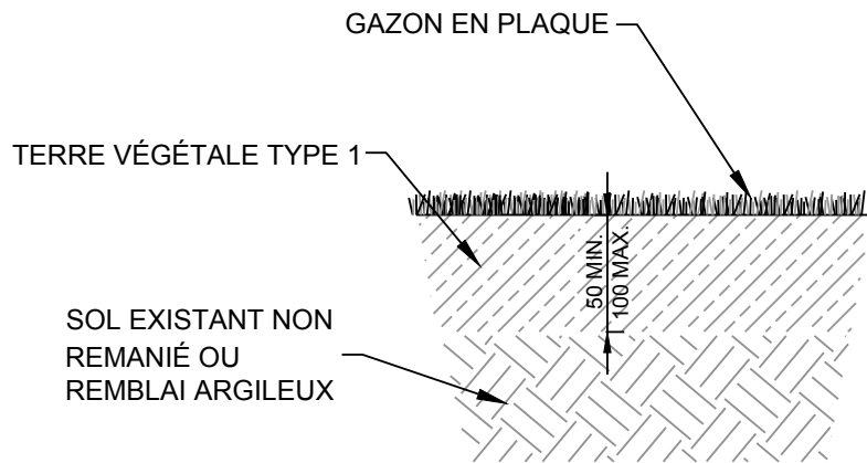
COUPE ENGAZONNEMENT
